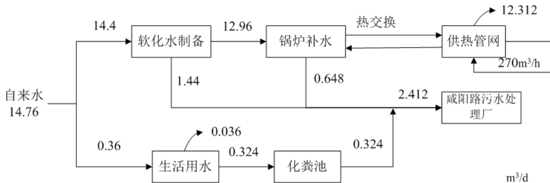
图2 本项目建成后锅炉房总水平衡图
