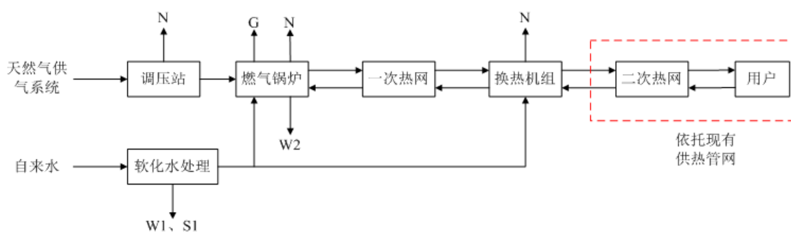
图7 本项目燃气锅炉运行流程及产污节点图
