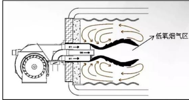
图8 低氮燃气器原理示意图
