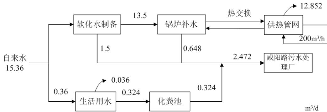
图5 现有项目水平衡图
